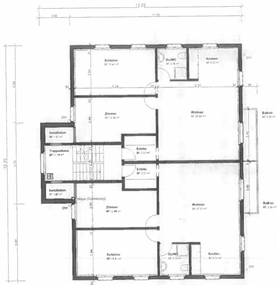
1./2. Obergeschoss
