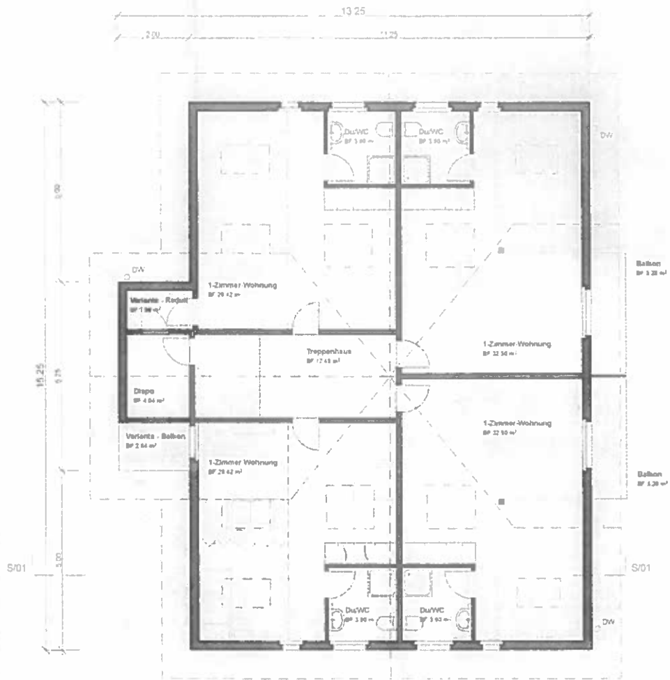
Dachgeschoss
